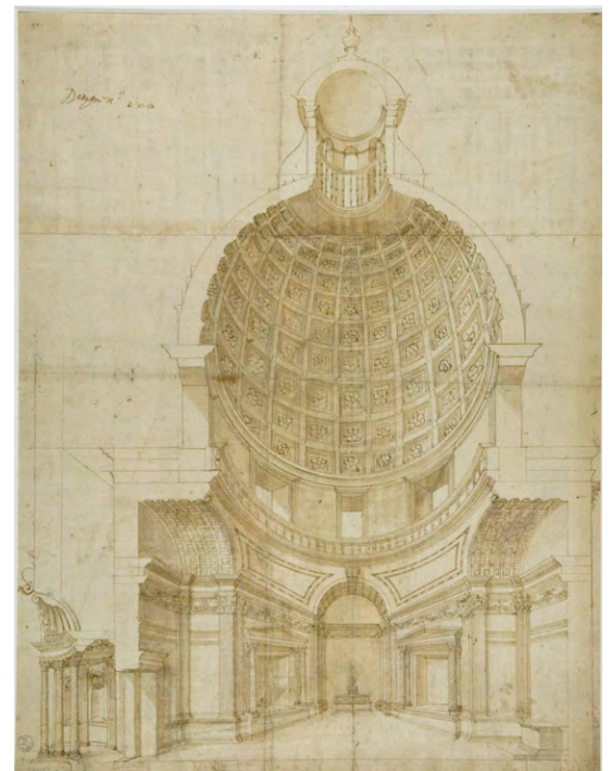
Alzato interno in prospettiva di una Chiesa o capella a croce greca Giamberti Giuliano dit Giuliano da Sangallo 1510-1515 Dessin sur papier, encre, crayon noir Gallerie degli Uffizi, Gabinetto dei Disegni e delle Stampe, Florence (Italie)
