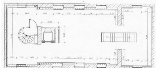
Premier étage
